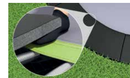
3 AkroSpring Pro System mit zusätzlicher Federschutzlasche
